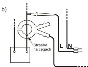
Sposób podłączenia cęgów
